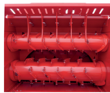
Double démêleurs Ø620+Ø460 à doigts fixes Brins courts, tous fourrages (entraînement mécanique)
