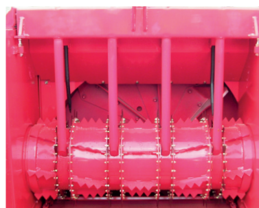
Simple démêleur Ø640 à doigts mobiles Brins longs, enrubannage (entraînement mécanique)
